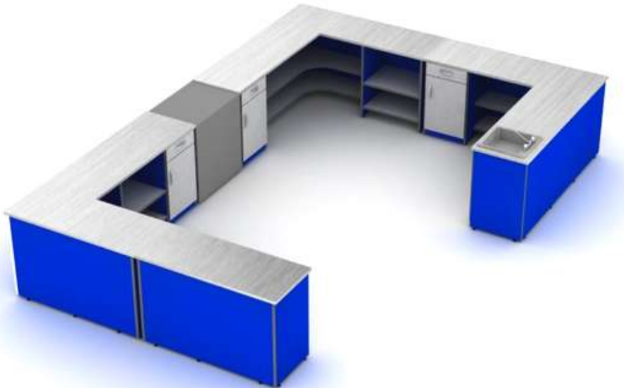
MÓDULO DE TRABAJO PARA LABORATORIO H 91.5 536 X 380 CM CUBIERTA ACERO INOX CON ÁREA DE TARJA 02.
