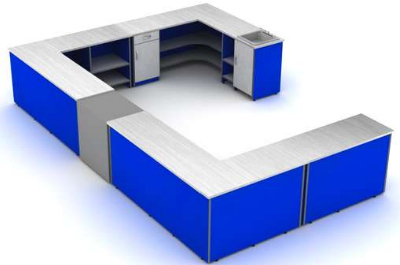
MÓDULO DE TRABAJO PARA LABORATORIO H 91.5 536 X 380 CM CUBIERTA ACERO INOX CON ÁREA DE TARJA 03.
